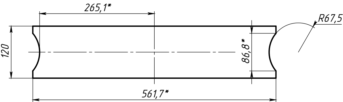
Поз.1 (Скоба) развертка
